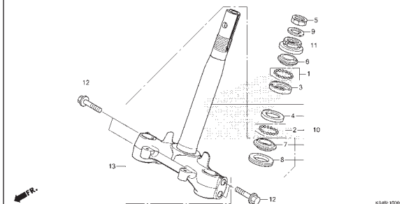
F-10 STEERING STEM
